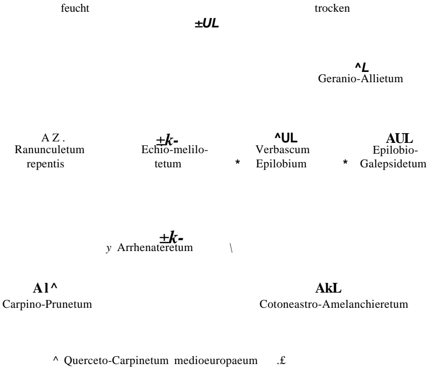
Abb. 2.1/1: Sukzessionsschema aufgelassener Weinbergflächen
